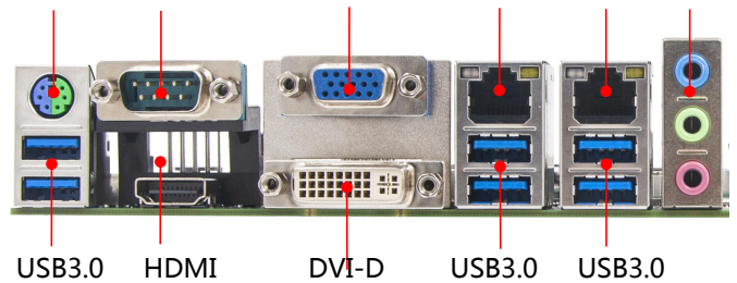
PS/2 COM1 VGA LAN LAN Audio
